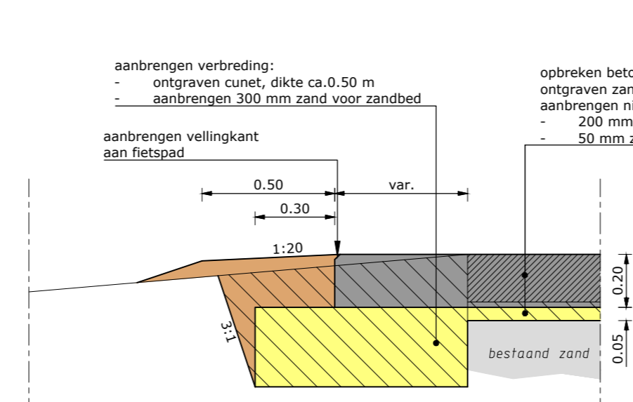
DETAIL 03: VERBREDING schaal 1:20
