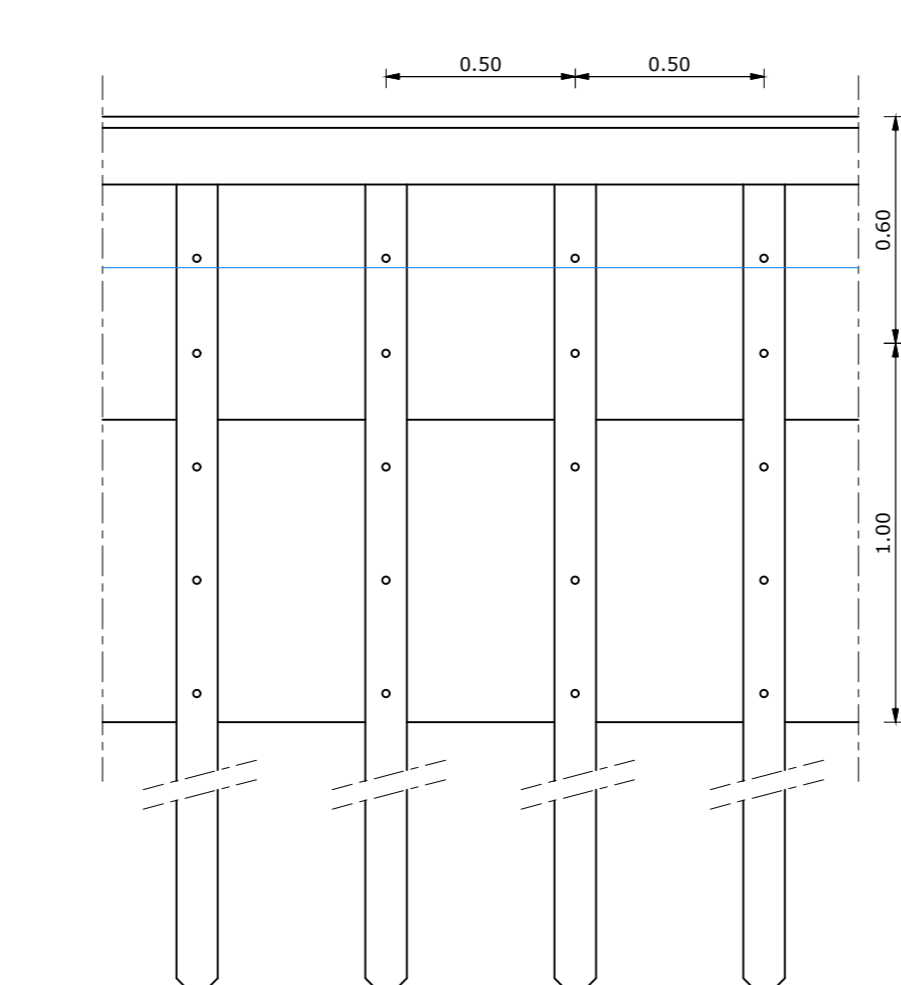
DETAIL 02: PAAL-SCHOT BESCHOEIING schaal 1:20
