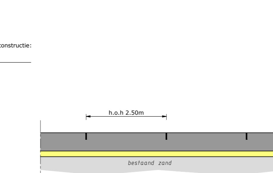
DETAIL 04: KRIMPVOEGEN schaal 1:20
