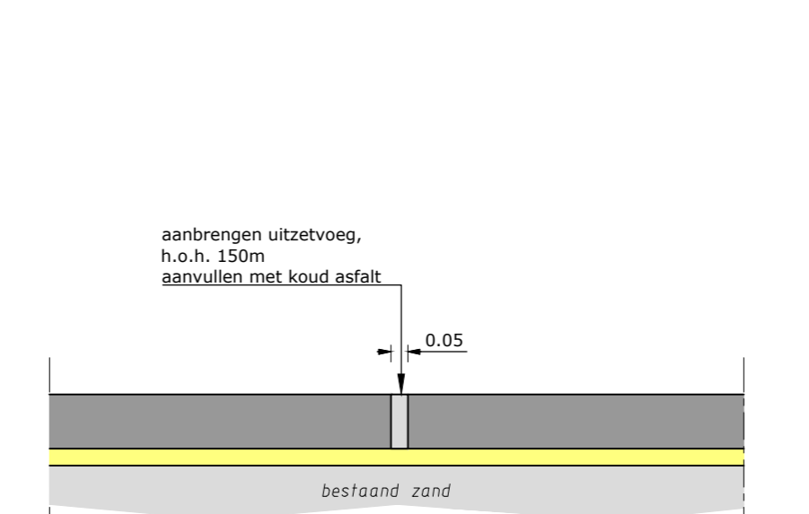
DETAIL 05: UITZETVOEG schaal 1:20
