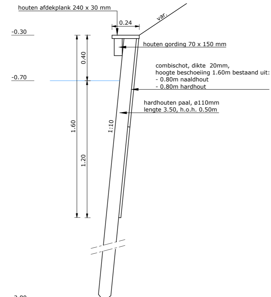
DETAIL 01: PAAL-SCHOT BESCHOEIING schaal 1:20
